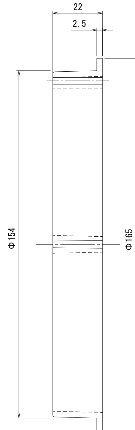
A-A断面図
