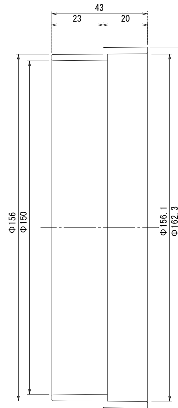
A-A' 断面図
